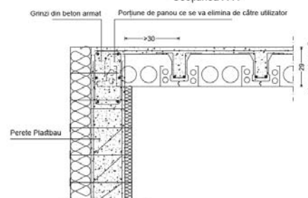
Secțiunea X-X
