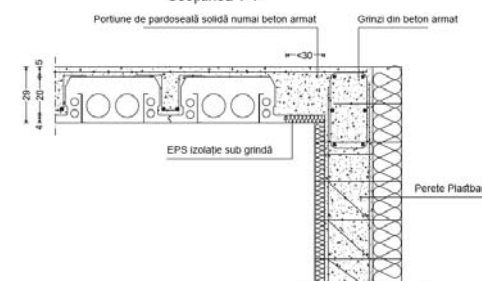
Secțiunea Y-Y
